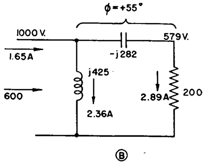
FIG. 2.27. Network B.
