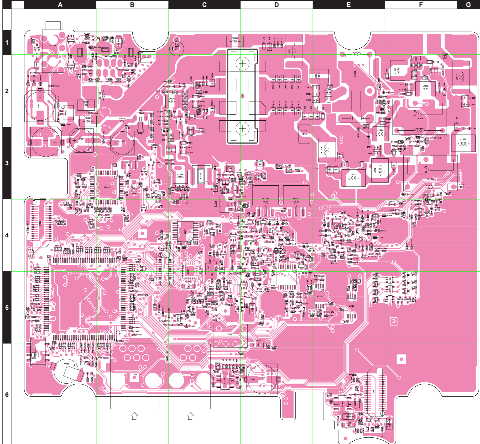
MAIN-2
