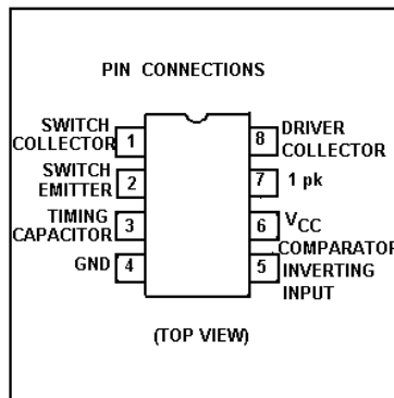
U2 +12 VOLT REGULATOR 19A134717P2
