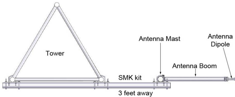
SMK-125-A3
