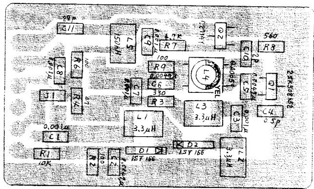
VCO (Part)
